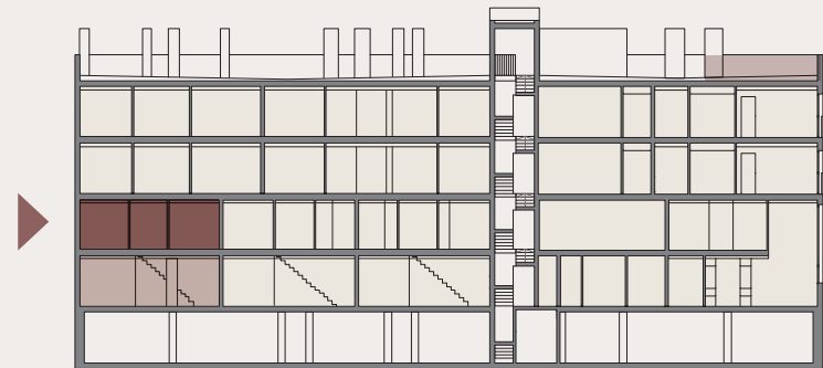
SECCIÓN: ALTILLO
